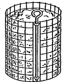
Drahtsilo ohne Plastikeinsatz für Sammelhaufen
